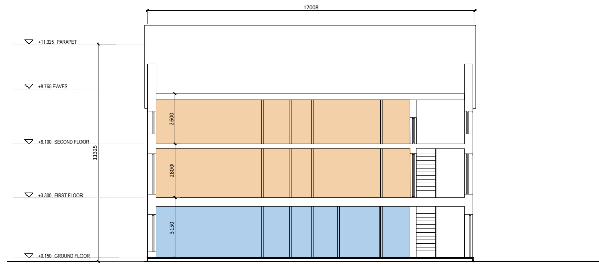
SECTION A-A 1:200
