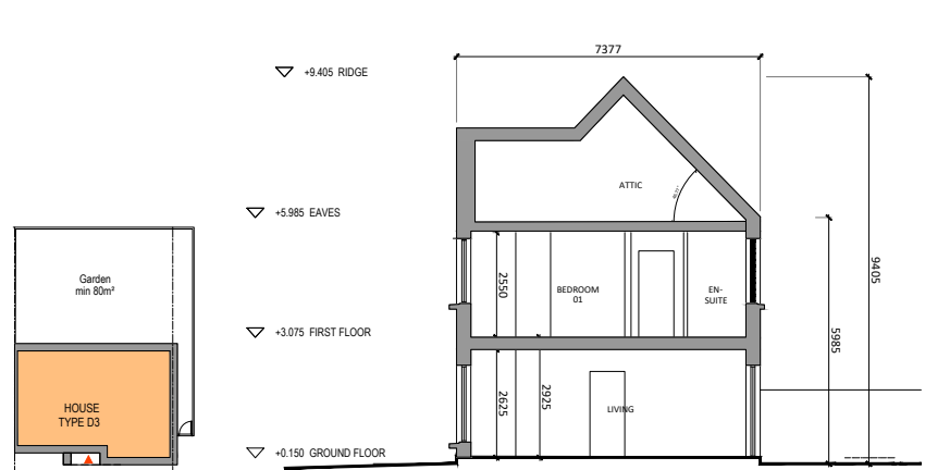
Section A-A 1:200
