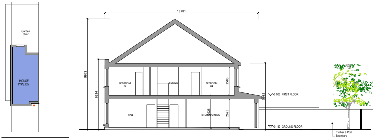
Section A-A 1:200
