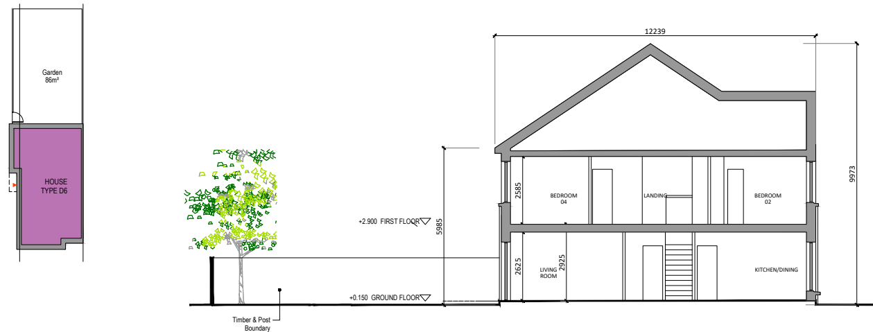
Section A-A 1:200
